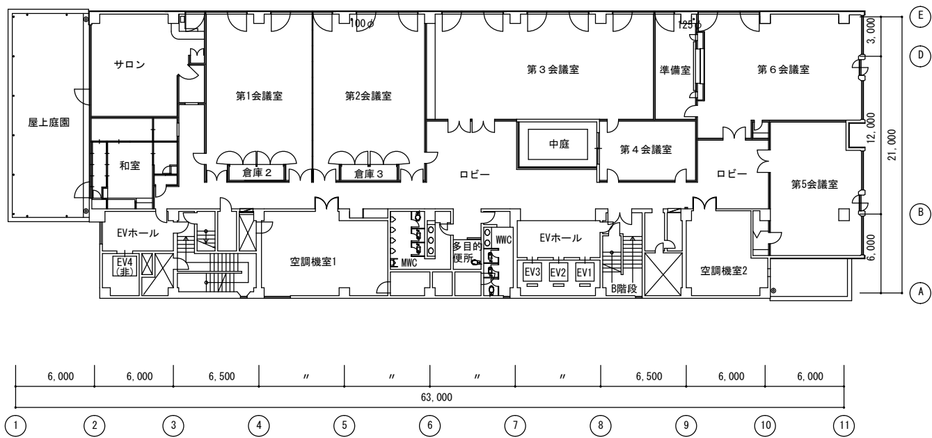
8階平面図 1 / 400
