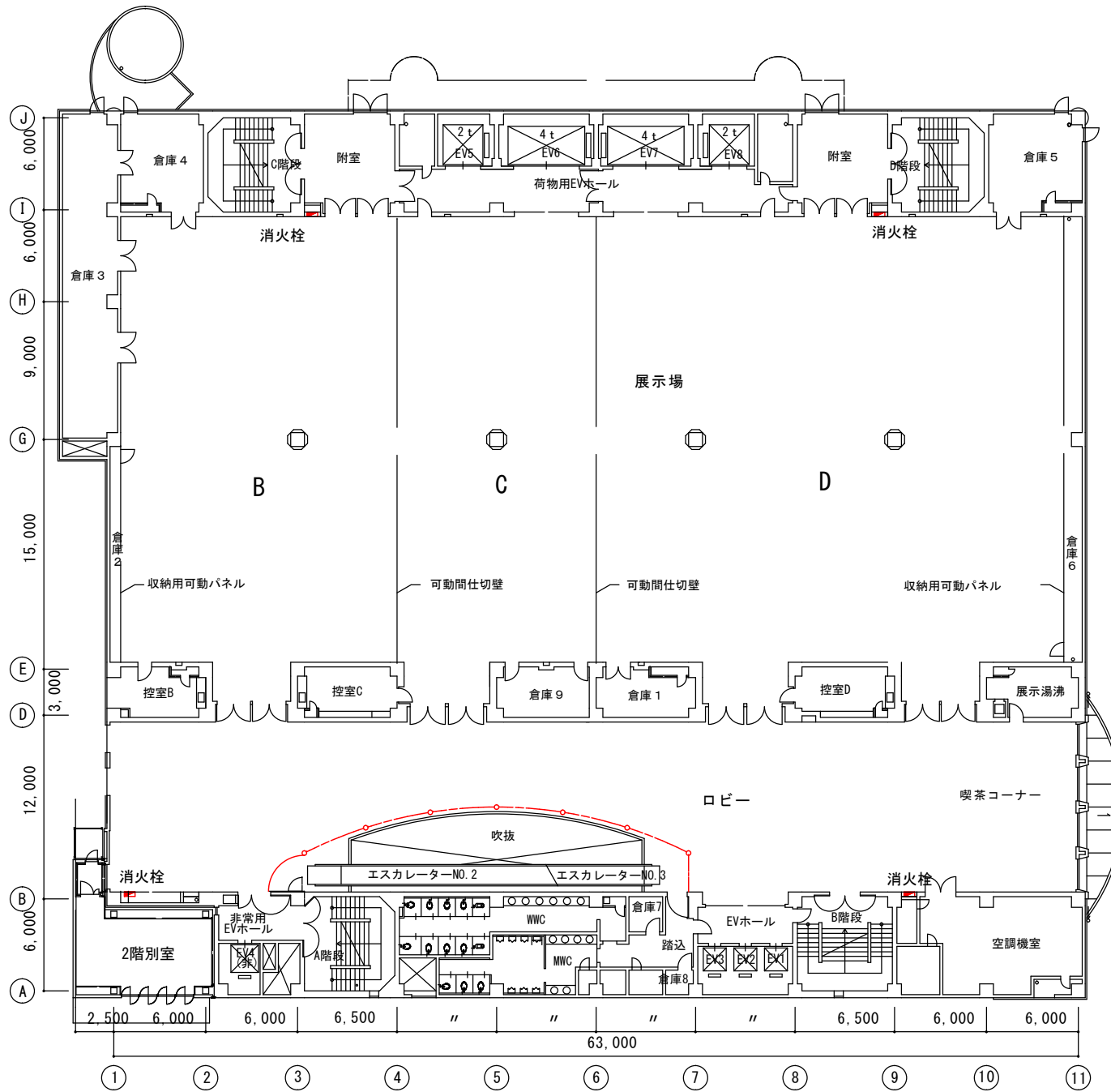
2階平面図 1/400
